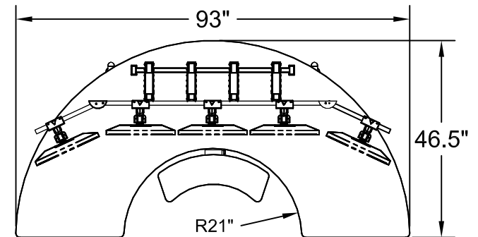
TOP VIEW SCALE: 3/8" = 1' - 0"
